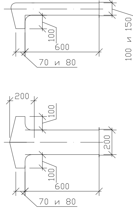
Вид элементов бортового отсоса двустороннего и одностороннего
